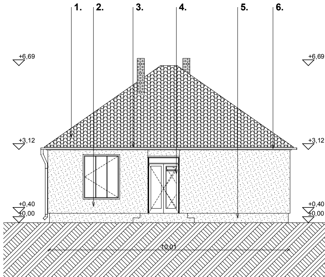
Nyugati-Homlokzat
