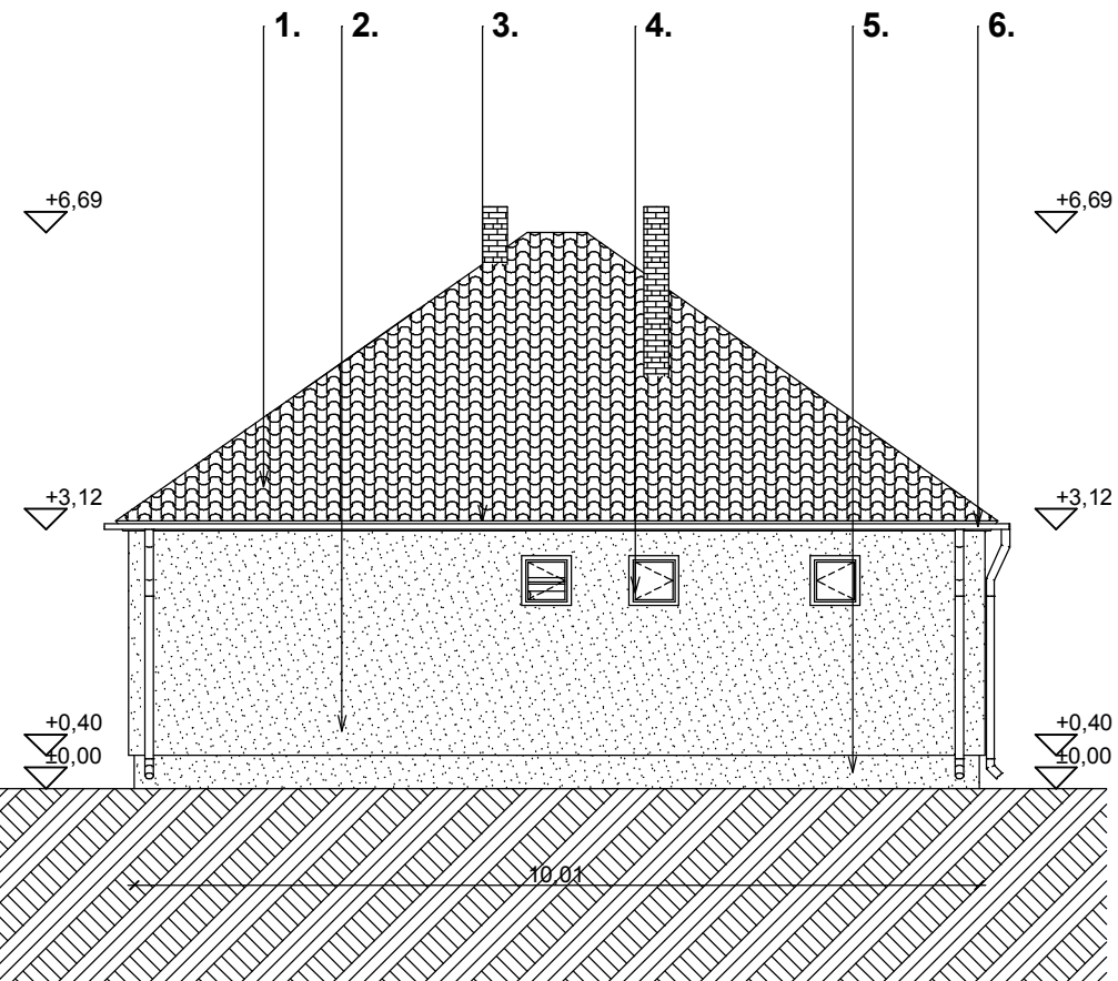
Keleti-Homlokzat
